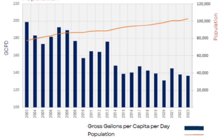
Gross Gallons per Capita per Day (GCPD) & Population
